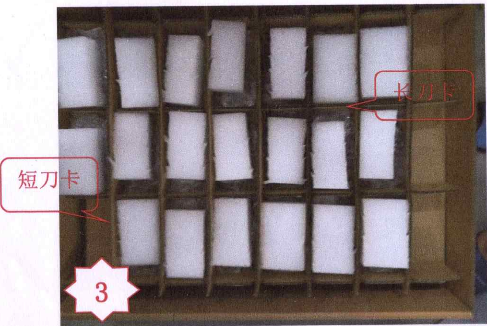
图三, 将 PA571 按照每层 120 个, 每箱三层的方式包装, 同时在底部和每层的顶部各放一块隔板, 共 4 块隔板。
